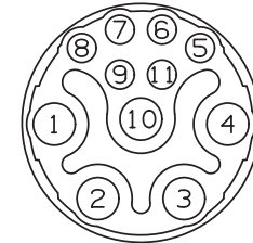
SOLDER LUG VIEW
