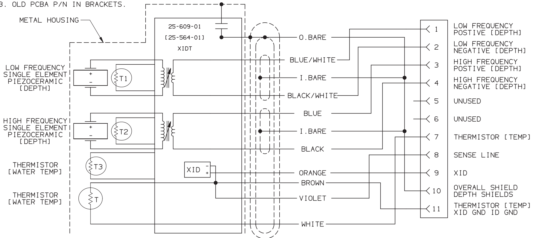
SOLDER LUG VIEW
