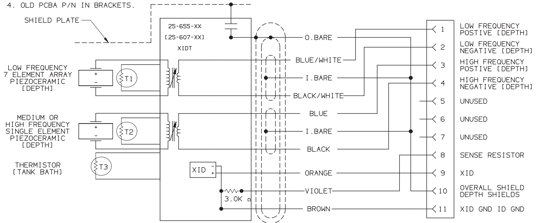
SOLDER LUG VIEW
